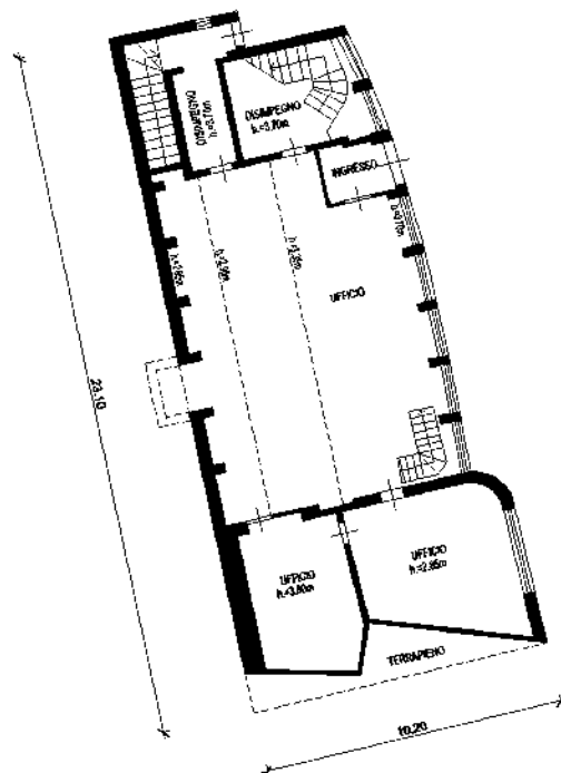
PIANOTERRA
