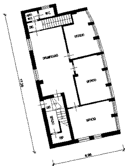
PRIMO PIANO h.=2.80m
