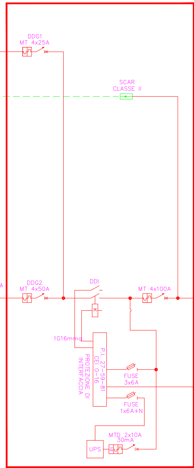
QUADRO LATO CORRENTE ALTERNATA
