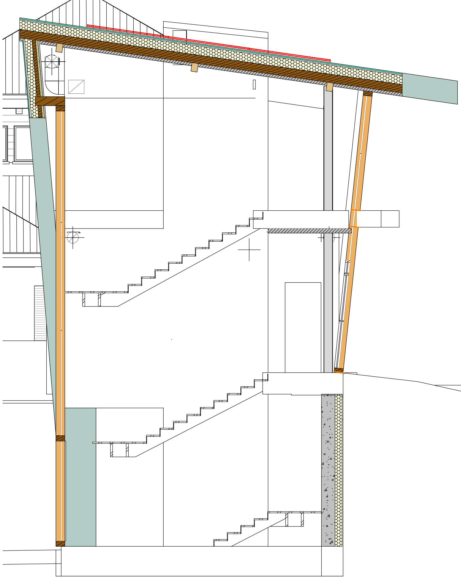
VISTA IN SEZIONE - SCALA 1:50
