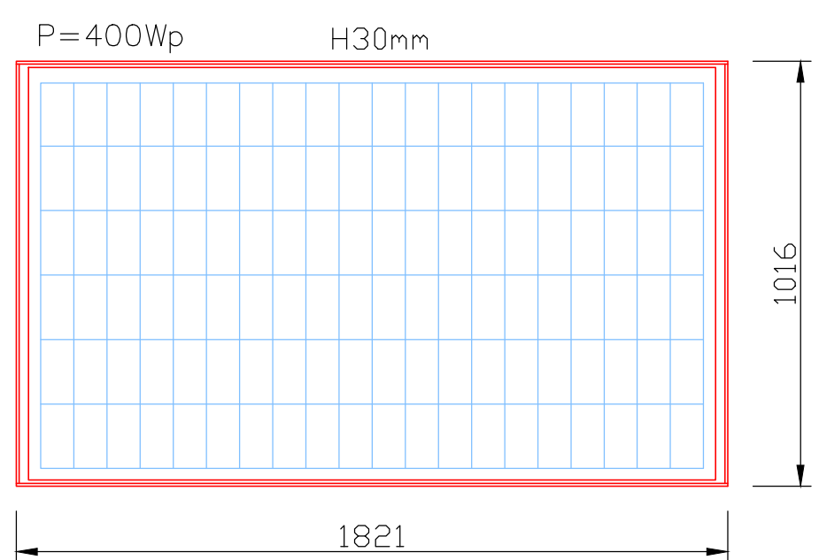
PARTICOLARE PANNELLO FOTOVOLTAICO
