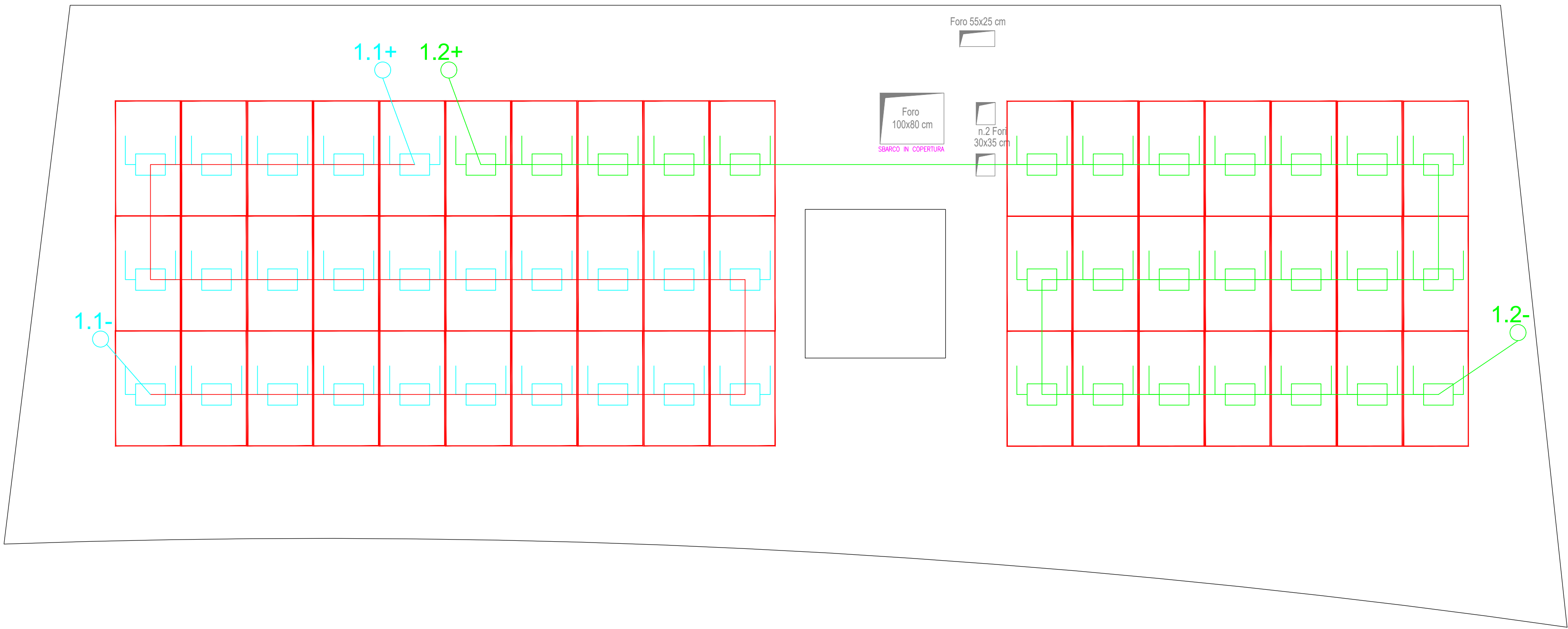
STRINGHE DI COLLEGAMENTO PANNELLI FOTOVOLTAICI - SCALA 1:50
