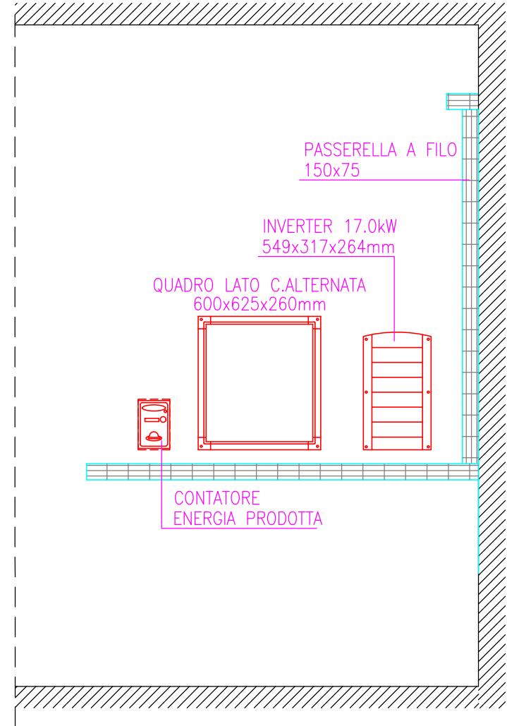
PARTICOLARE INSTALLAZIONE QUADRO LATO C.ALTERNATA ED INVERTER
