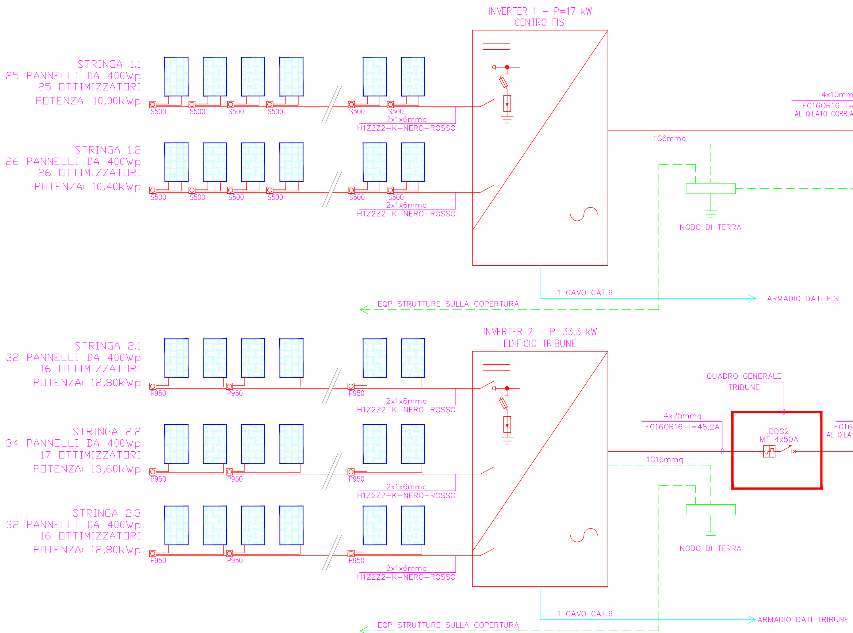
SCHEMA UNIFILARE IMPIANTO FOTOVOLTAICO CENTRO FISI ED EDIFICIO TRIBUNE
