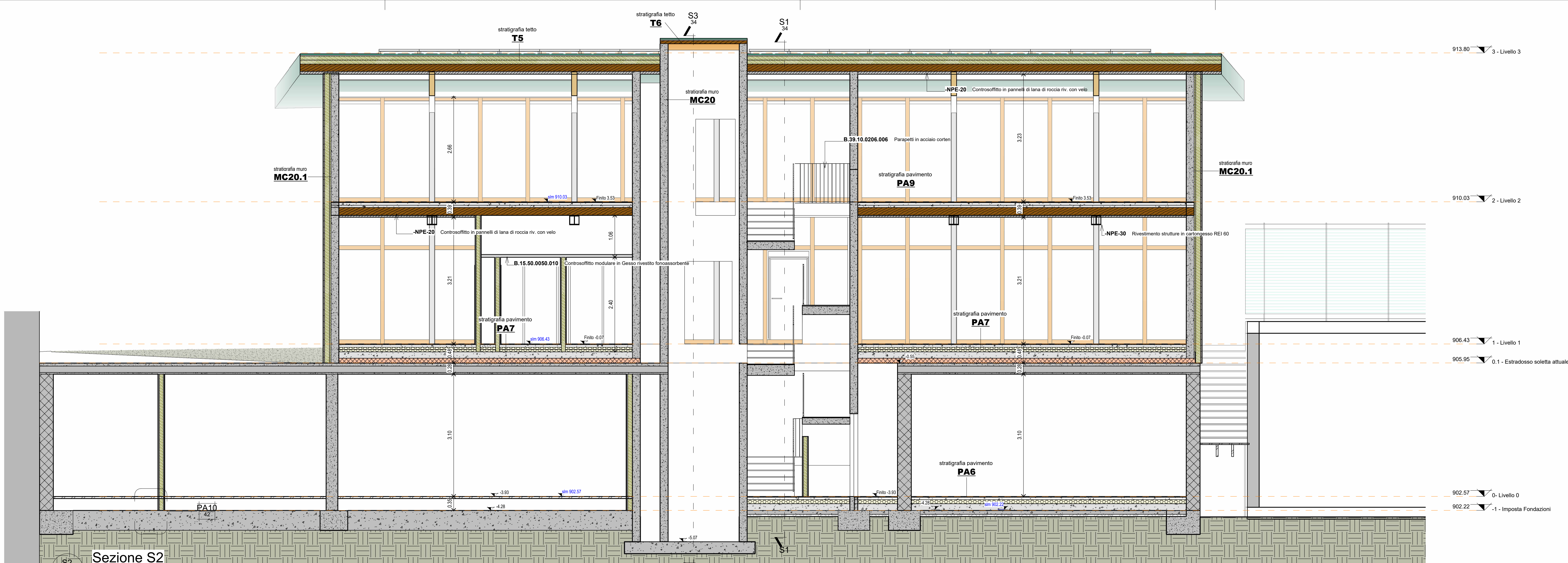
Sezione S2 Sezione progetto 1 : 50
