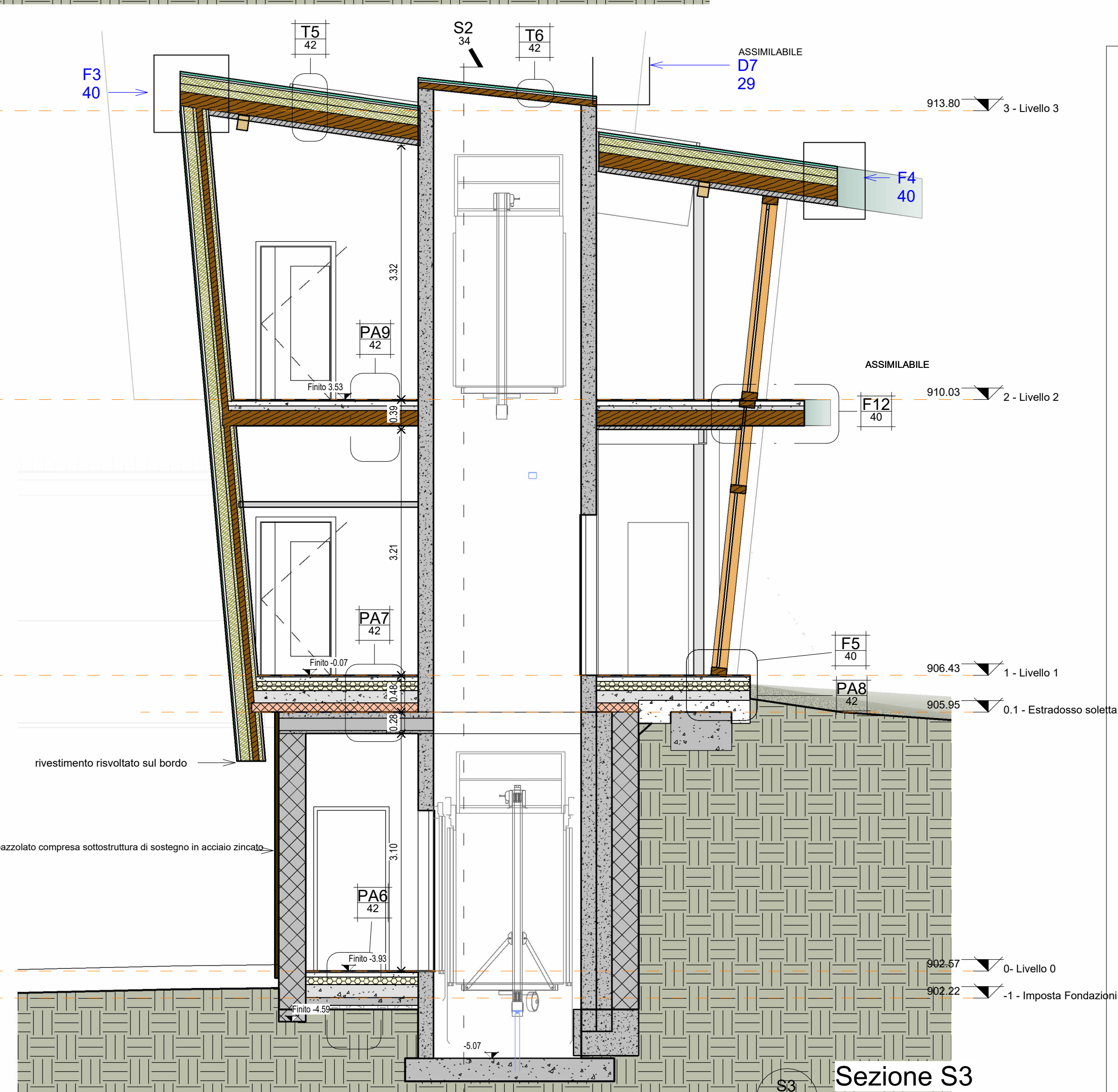
Sezione S3 Sezione progetto 1 : 50
