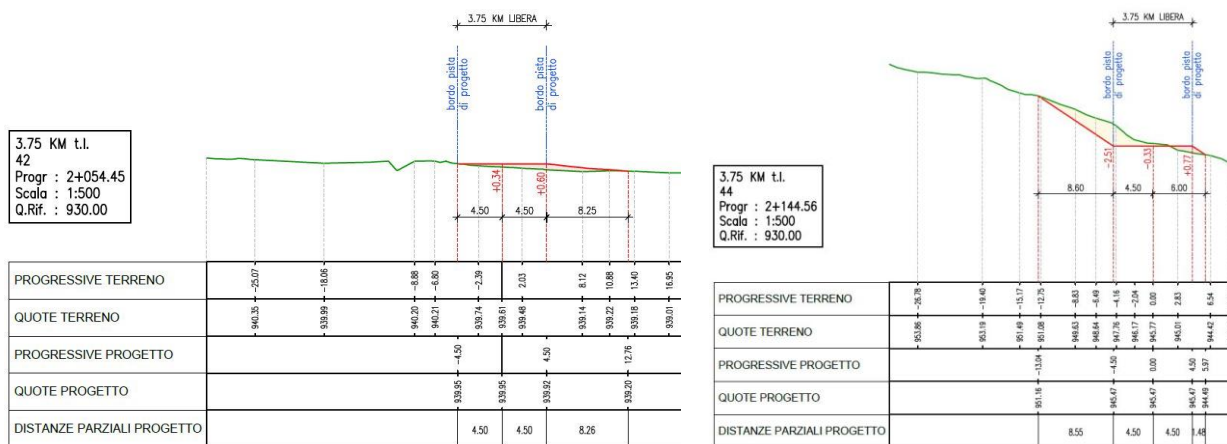
Figura 8: Estratto sezioni - scala a vista
