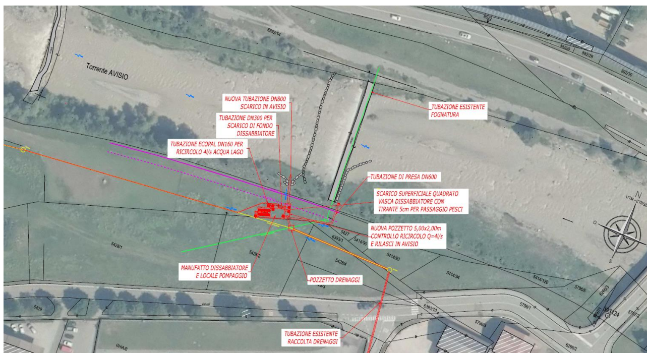
Figura 19: Inquadramento della nuova opera di presa su estratto C.C. Tesero
