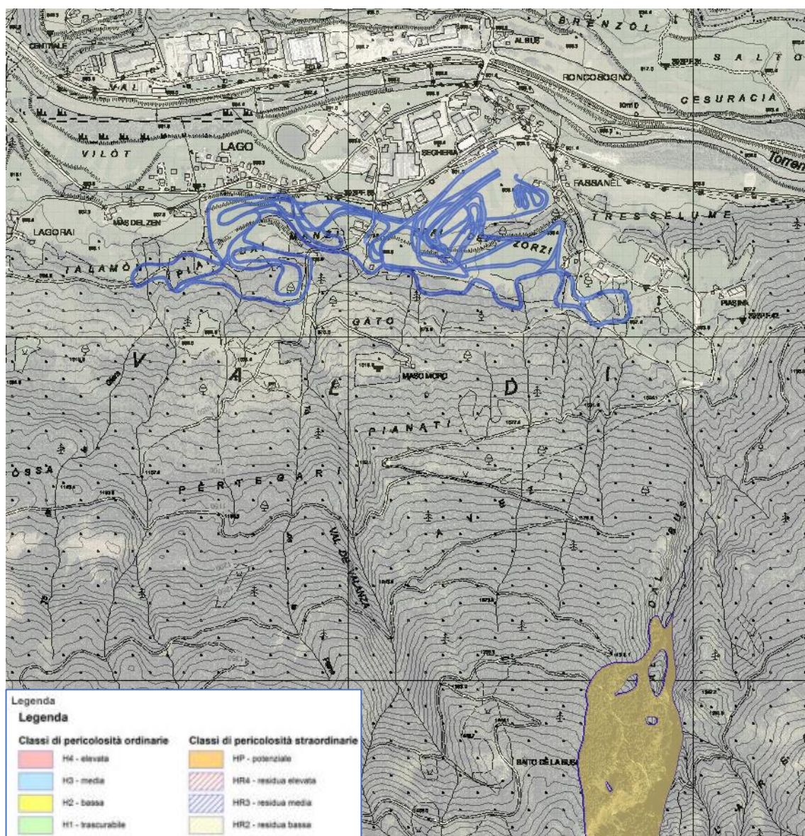
Figura 2.1: Estratto della Carta della Pericolosità Valanghiva per l'area oggetto di studio.
