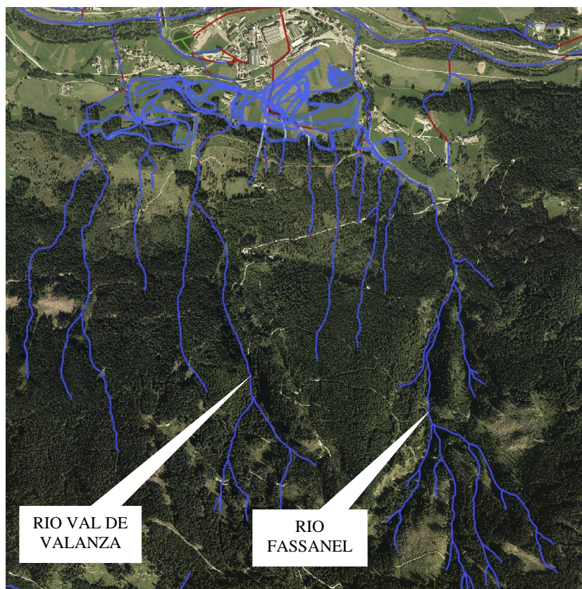
Figura 3.1: Principali corsi d’acqua che interessano l’area delle piste del Centro del Fondo.
