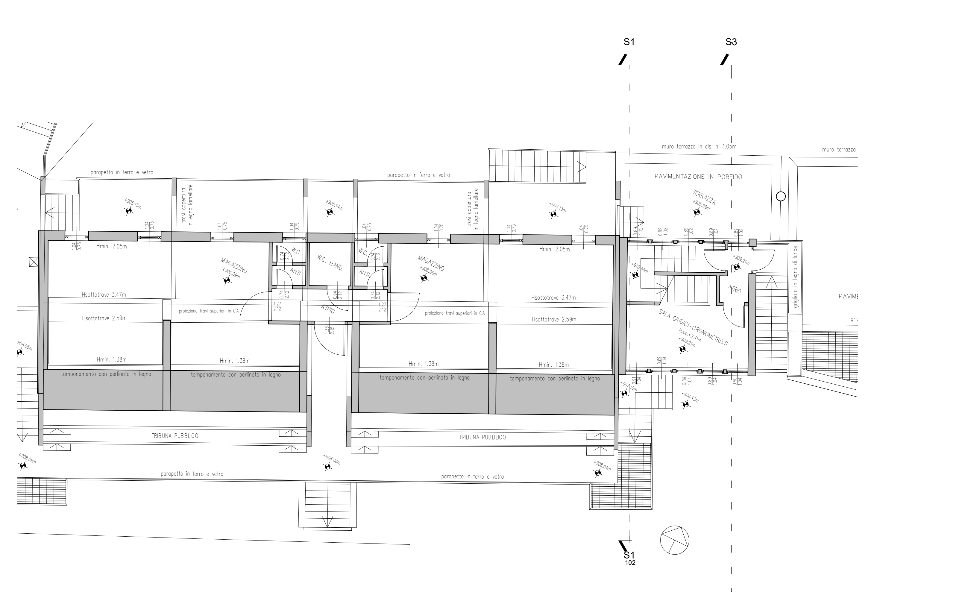
3 101 Pianta Piano Primo 1 : 100
