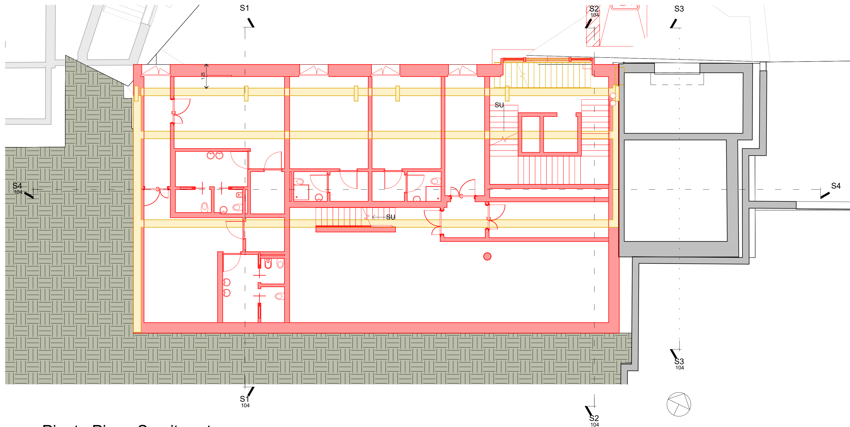
1 103 Pianta Piano Semiterreno 1 : 100
