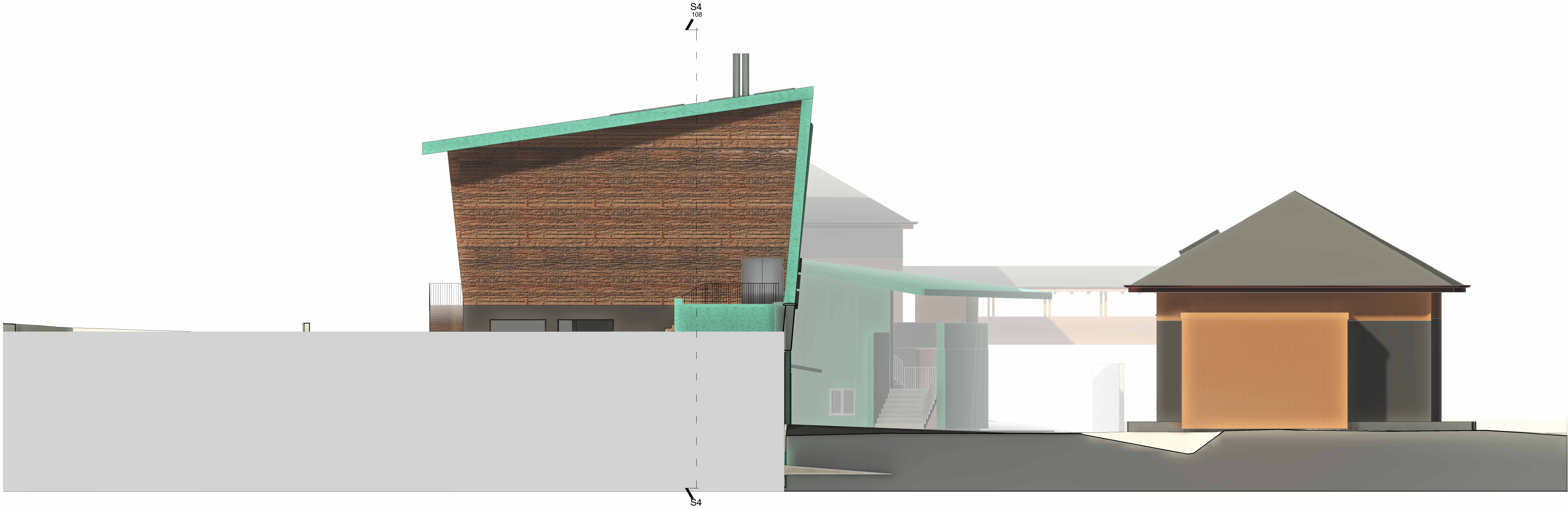
2 110 Prospetto Est 1 : 100
