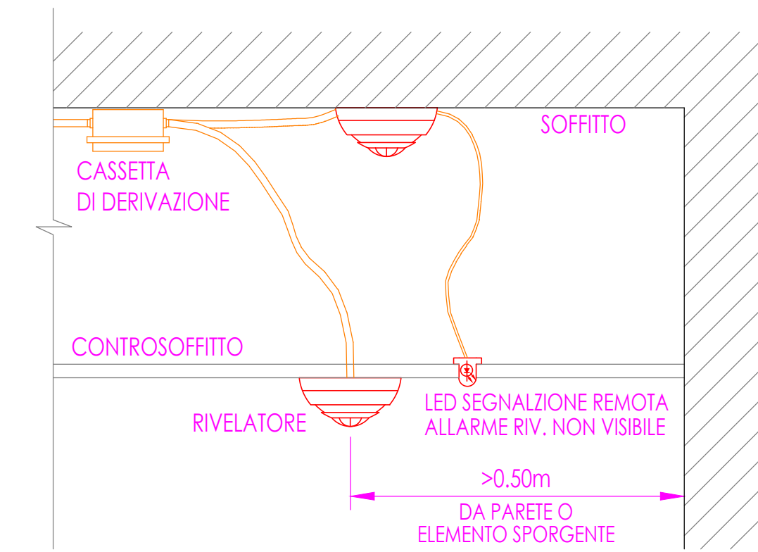
PARTICOLARE INSTALLAZIONE RILEVATORE DI FUMO
